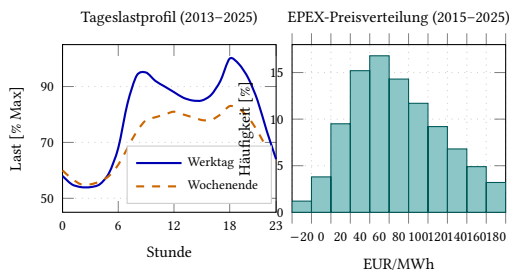
Abbildung 1: Links: mittleres Tageslastprofil für Werktag und Wochenenden (normiert auf das Tagesmaximum der Werktage). Rechts: Verteilung der EPEX-Day-Ahead-Stundenpreise 2015–2025; der Median liegt bei ≈65 EUR/MWh, rund 4 % der Werte sind negativ.
