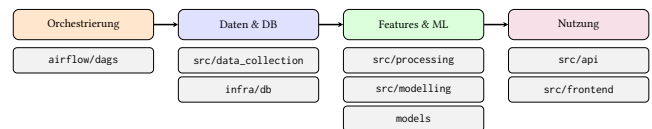
Abbildung 3: Projektstruktur: Die Ordner spiegeln den Datenfluss von Orchestrierung über Speicherung und Modellierung bis zur API und zum Dashboard wider.
