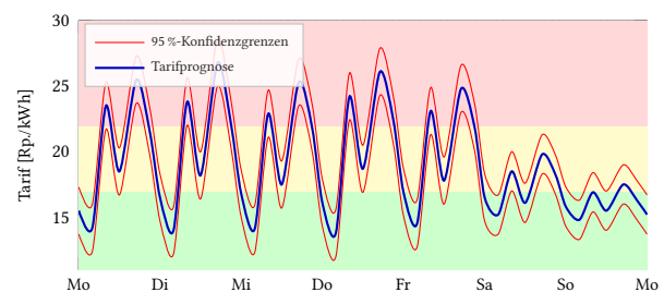
Abbildung 5: Beispielhafte 7-Tage-Tarifprognose mit Ampelzonen (grün \leq 17 , gelb 17–22, rot \geq 22 Rp./kWh) und 95%-Konfidenzband. Deutlich erkennbar: morgendliche und abendliche Preisspitzen an Werktagen sowie ein ruhigeres Wochenende (Sa/So).
