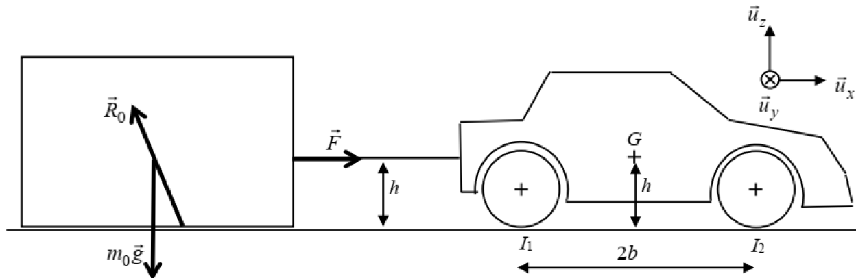
Figure 2 - Schéma de l'ensemble {container, filin, voiture}
