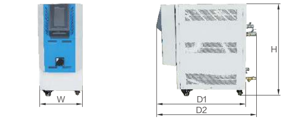
外型尺寸图 Dimensions 单位/Unit : mm
