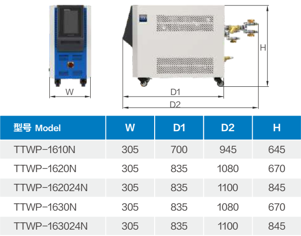
外型尺寸图 Dimensions 单位/Unit : mm
