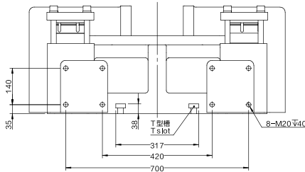
机械手安装孔位 Robot installation dimension
