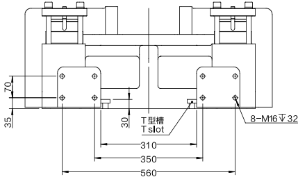
机械手安装孔位 Robot installation dimension
