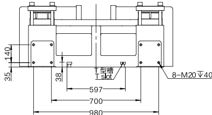
机械手安装孔位 Robot installation dimension
