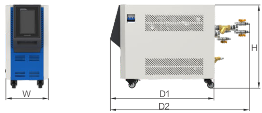
外型尺寸图 Dimensions 单位/Unit : mm
