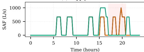
(d) Supply Air Flow
