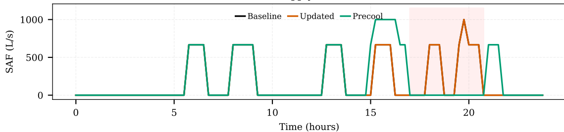
(d) Supply Air Flow
