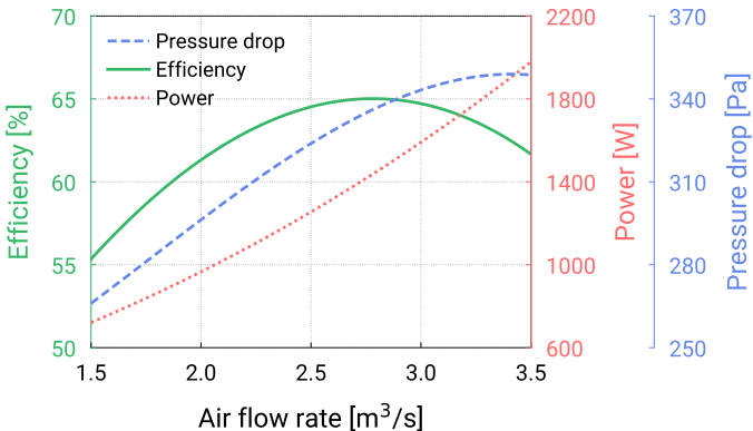
(b) Outdoor unit fan
