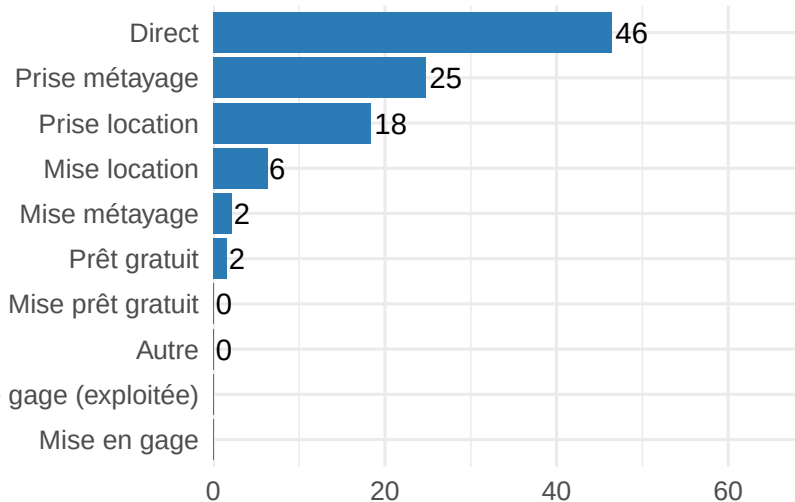
Marovoay
