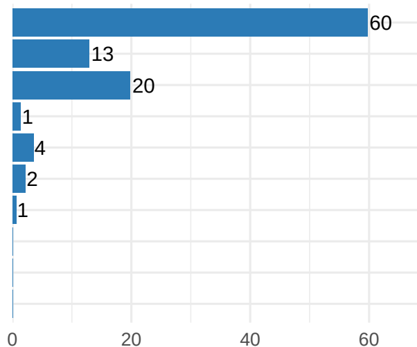
Alaotra
