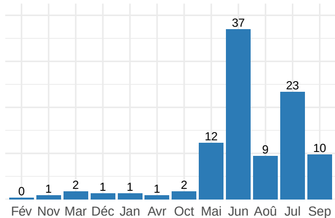
Alaotra
