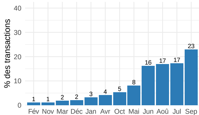
Marovoay
