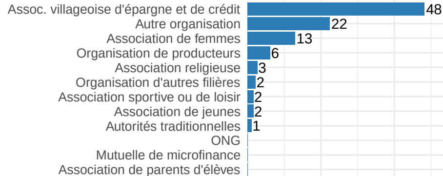
Marovoay
