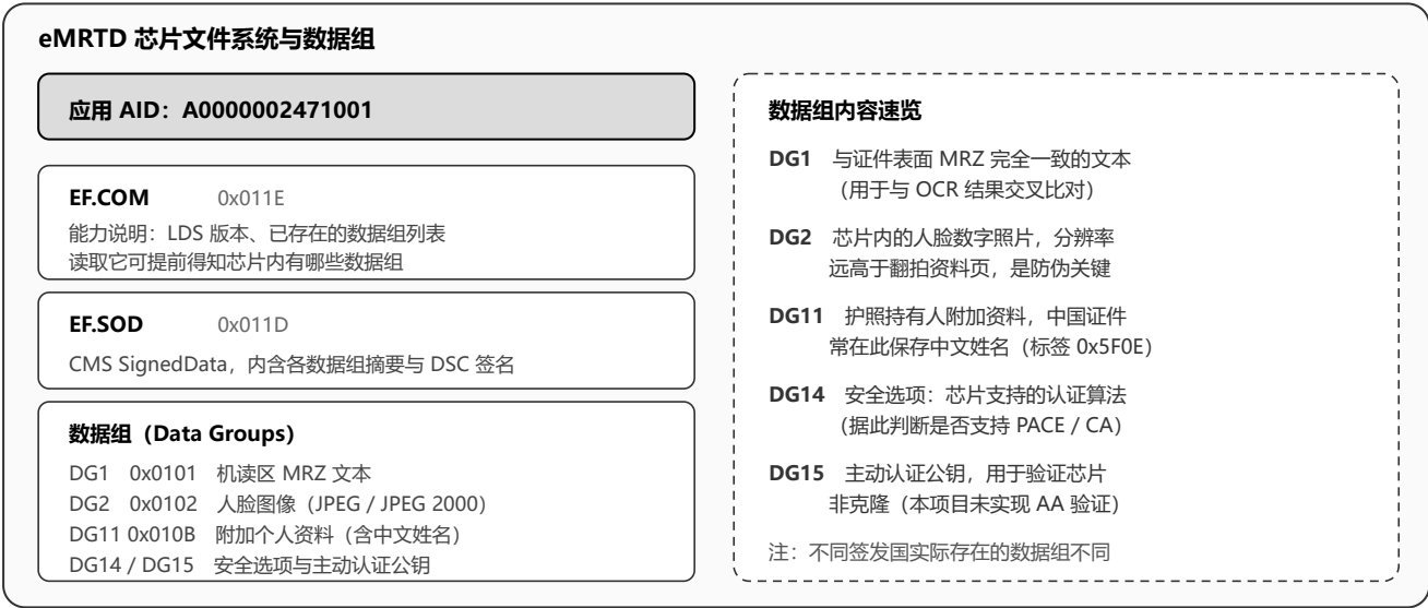
图 3-4 芯片文件系统结构与主要数据组
