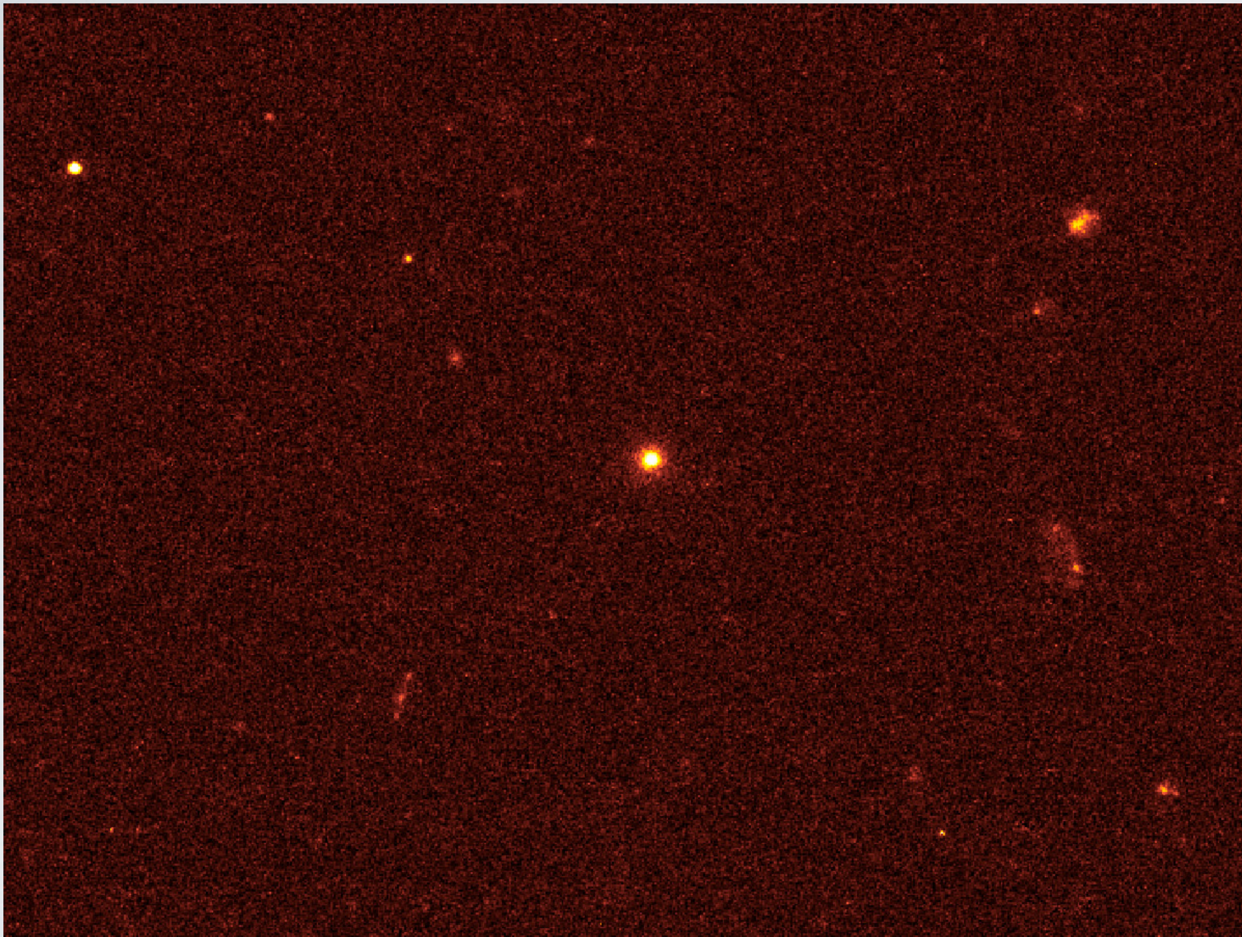
Swift J1644+57
