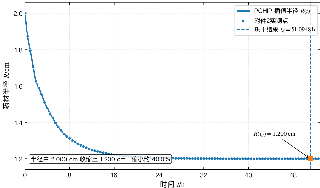
药材半径随烘干时间的变化
