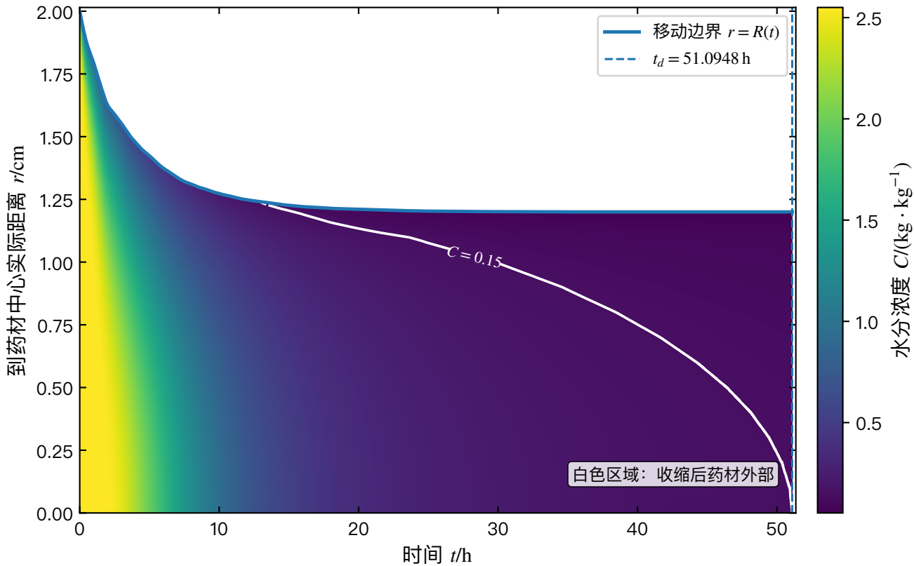
移动边界下药材内部水分浓度时空分布
