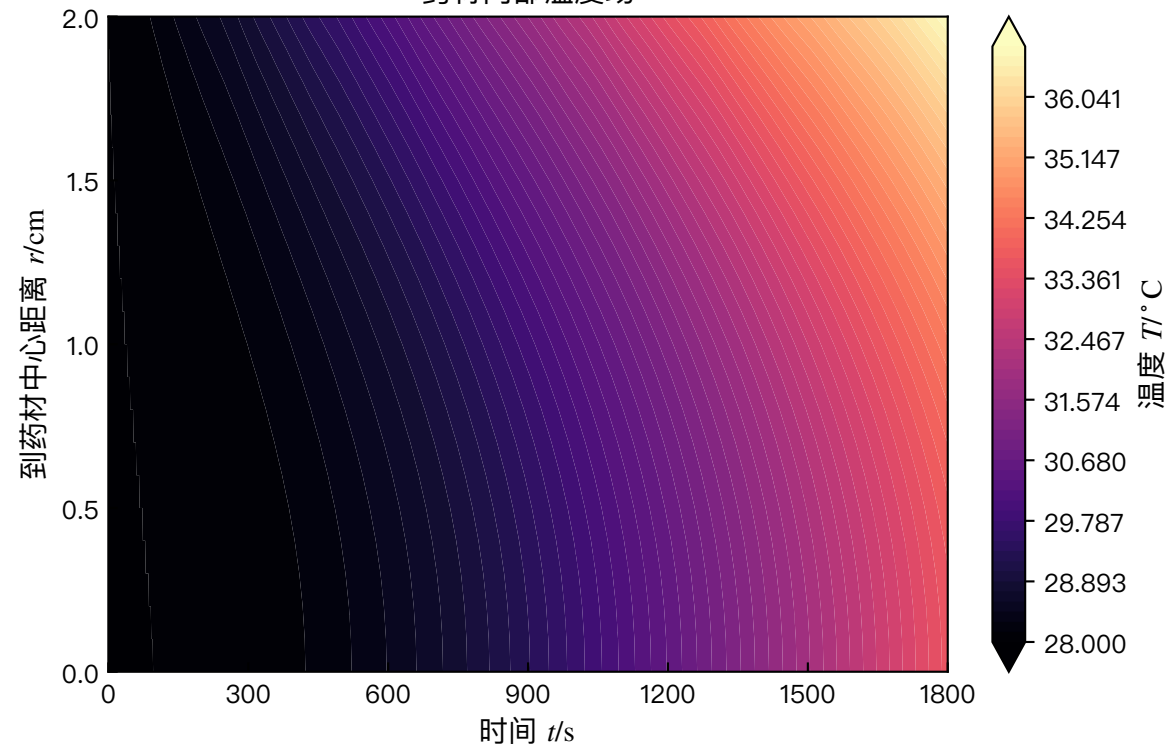
药材内部温度场
