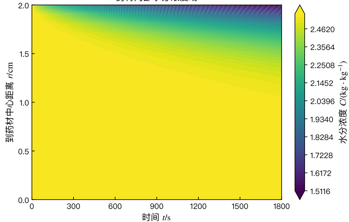
药材内部水分浓度场
