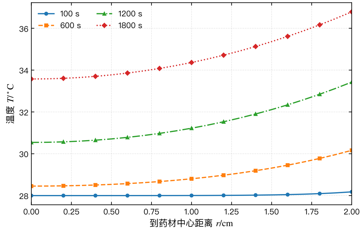
典型时刻温度径向分布
