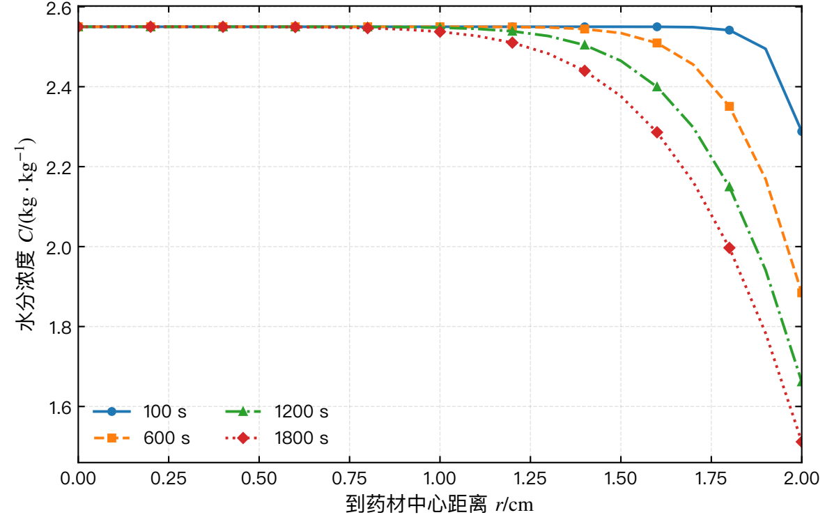
典型时刻水分浓度径向分布
