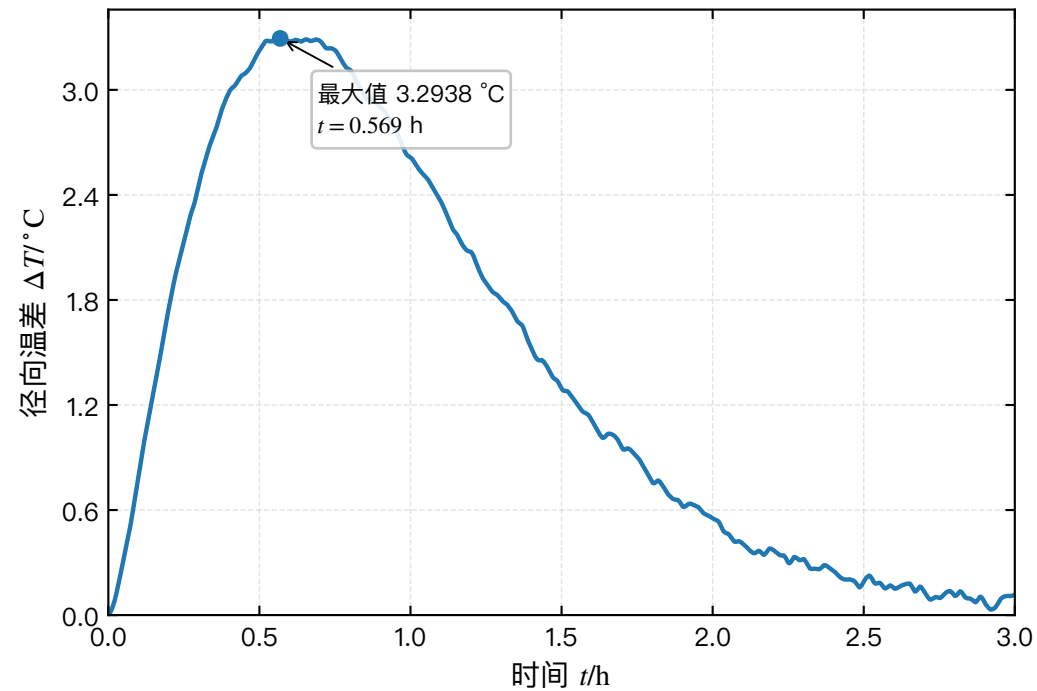
中心—表面径向温差
