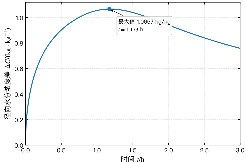
中心—表面水分浓度差
