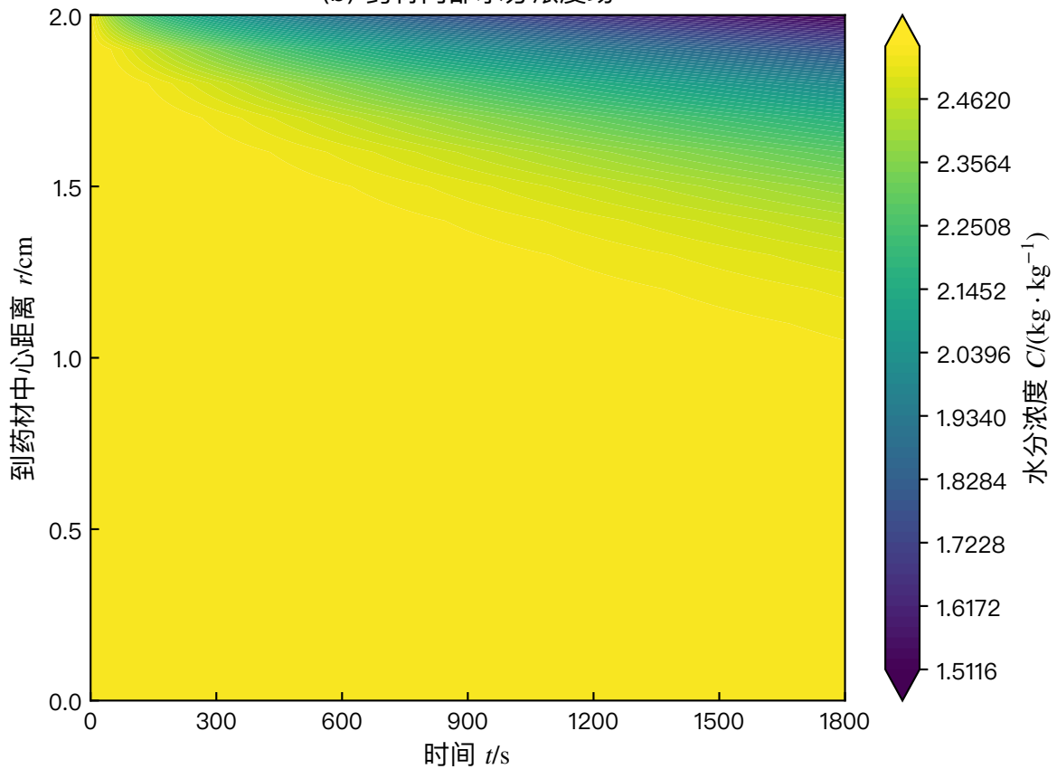
(b) 药材内部水分浓度场
