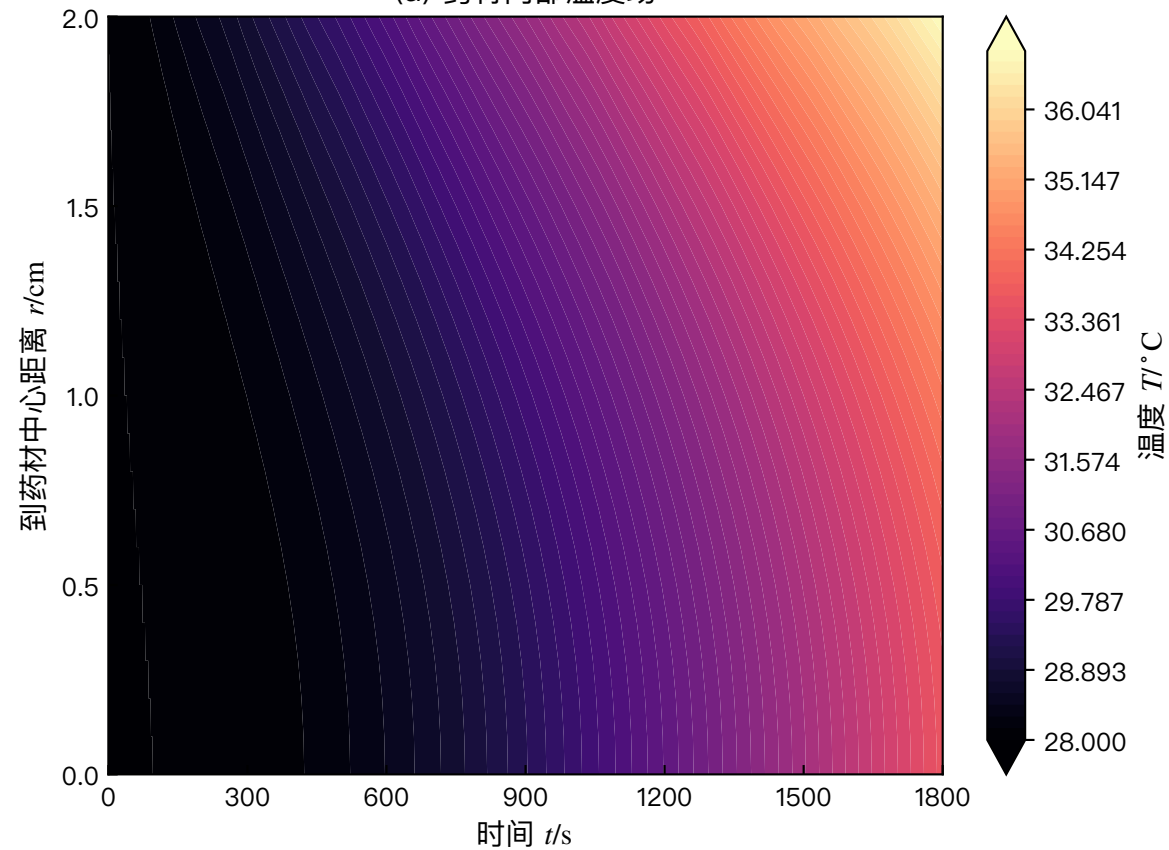
(a) 药材内部温度场
