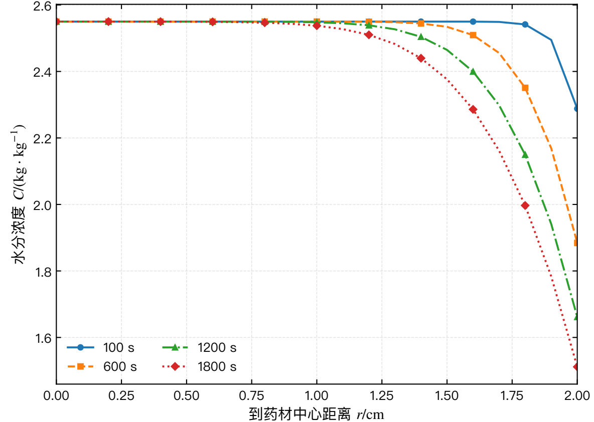
(b) 典型时刻水分浓度径向分布
