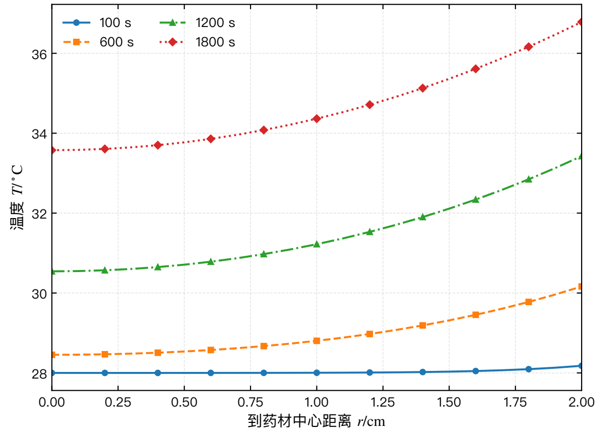
(a) 典型时刻温度径向分布
