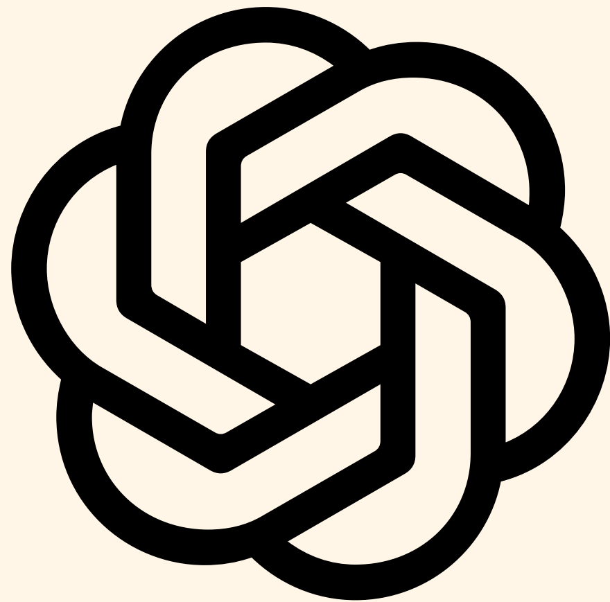
ChatGPT
