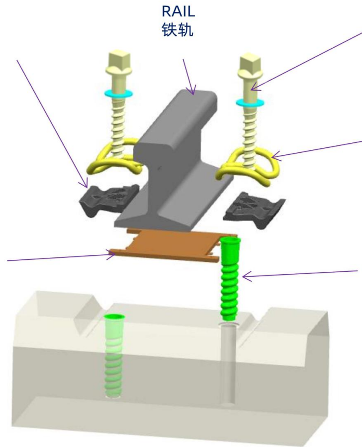
ANGLE GUIDE PLATES 轨距挡板
