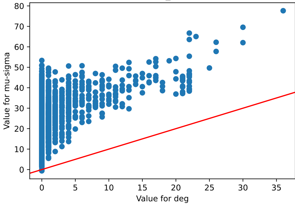
deg v/s mu-sigma Lung_73
