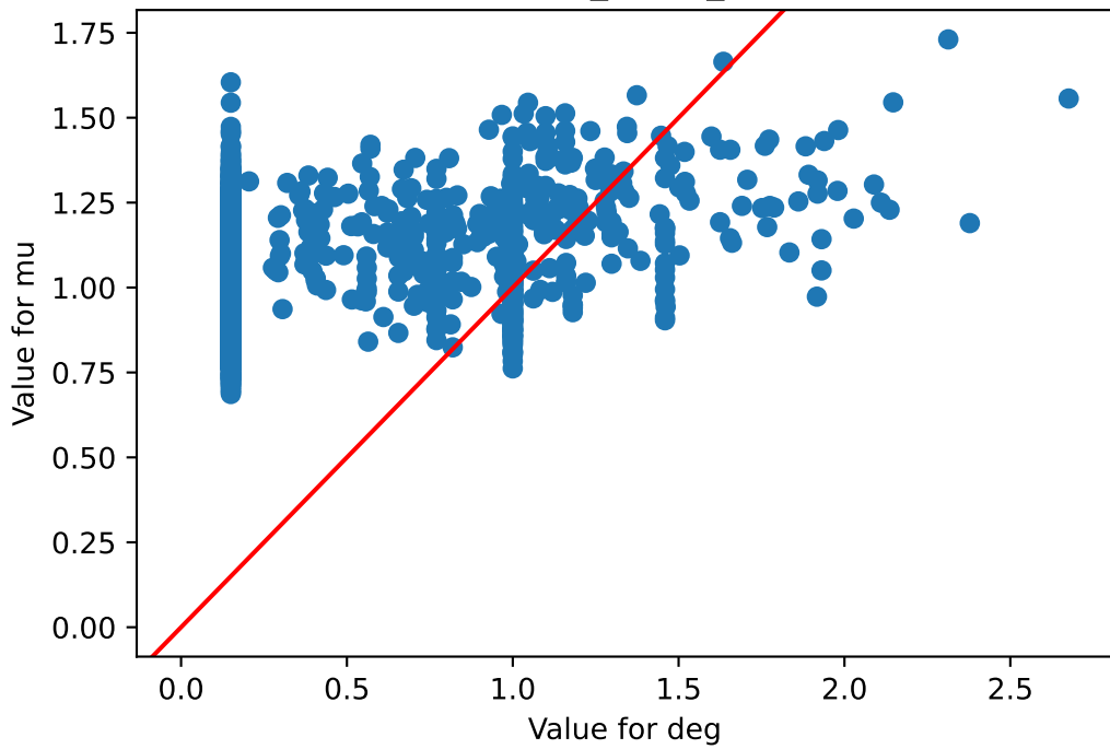
deg v/s mu Whole_Blood_73
