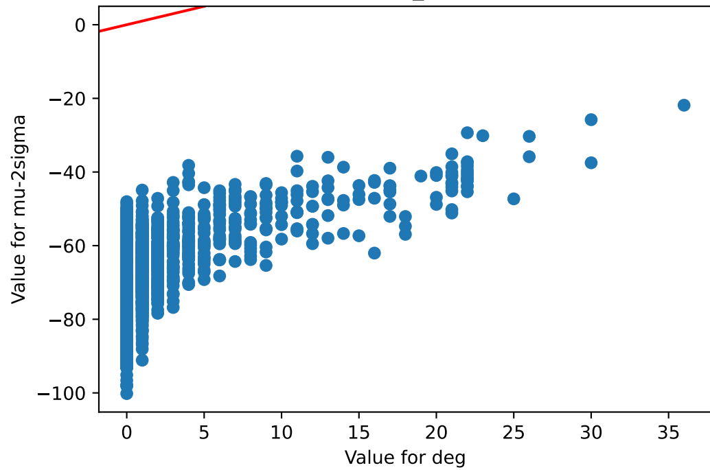
deg v/s mu-2sigma Lung_73
