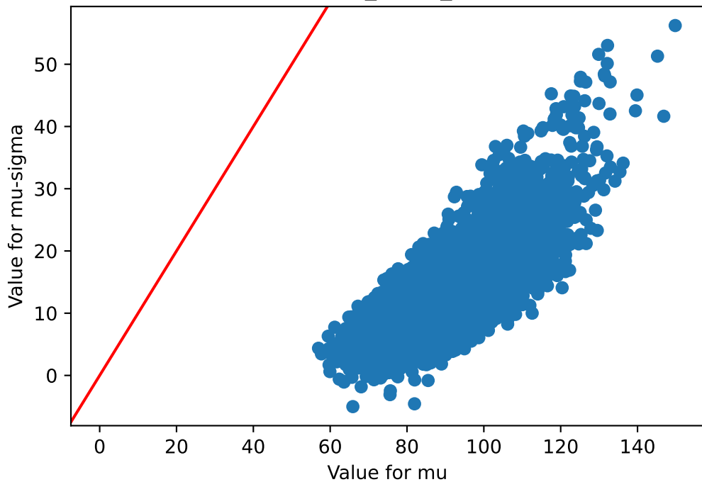
mu v/s mu-sigma Whole_Blood_73
