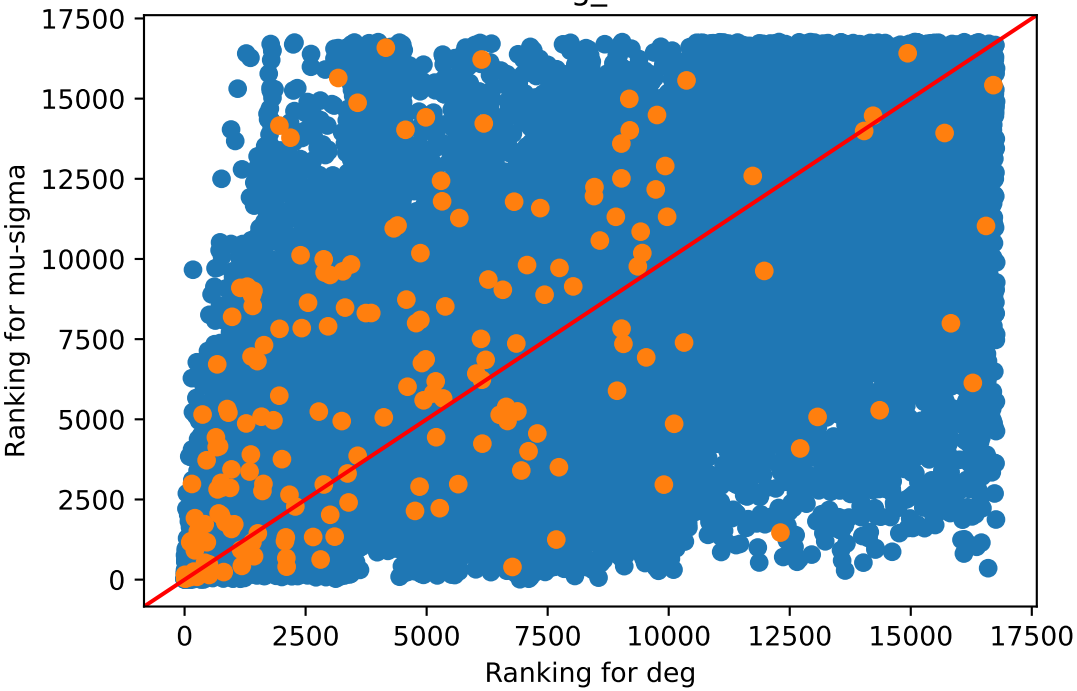
deg v/s mu-sigma Lung_237
