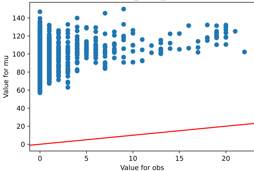
obs v/s mu Whole_Blood_73
