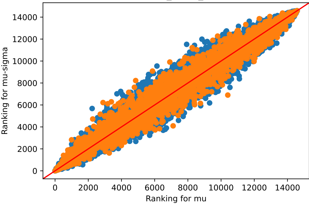
mu v/s mu-sigma Whole_Blood_73
