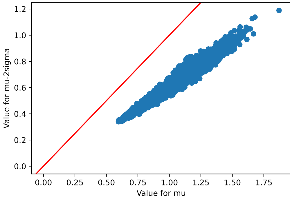
mu v/s mu-2sigma Lung_237
