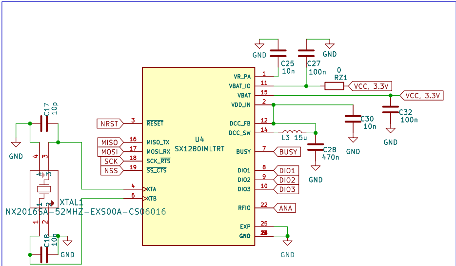
LoRa WAN Module
