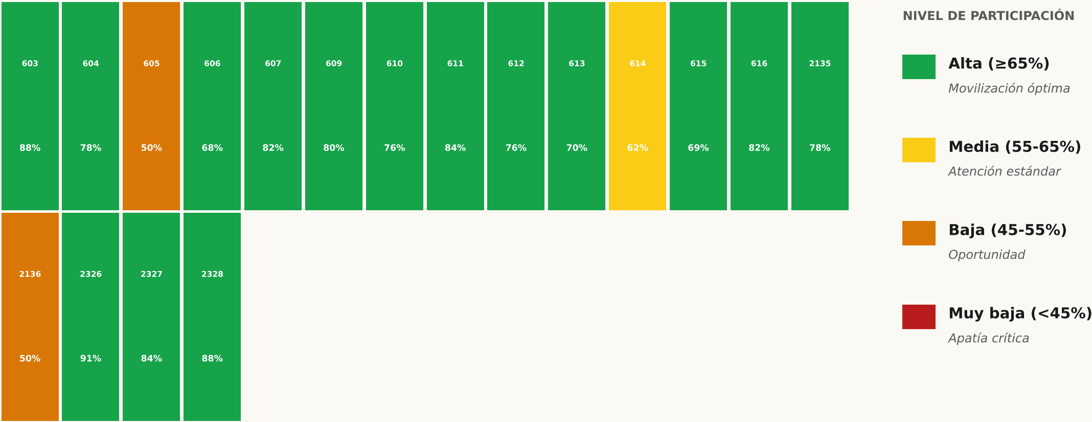
Distribución de 18 secciones electorales (cada celda = 1 sección)
