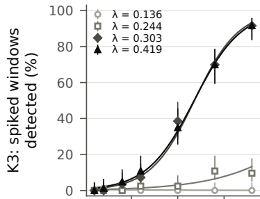
Hénon map
