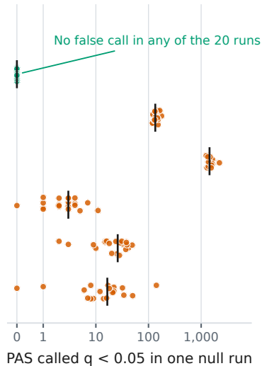
b False calls per null run
