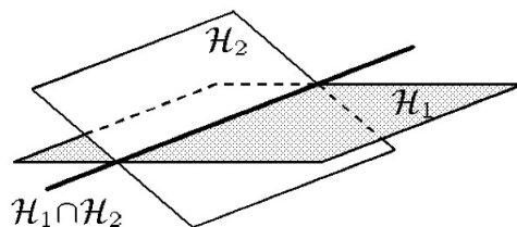
Рис. 3: Пересечение линейных подпространств.
