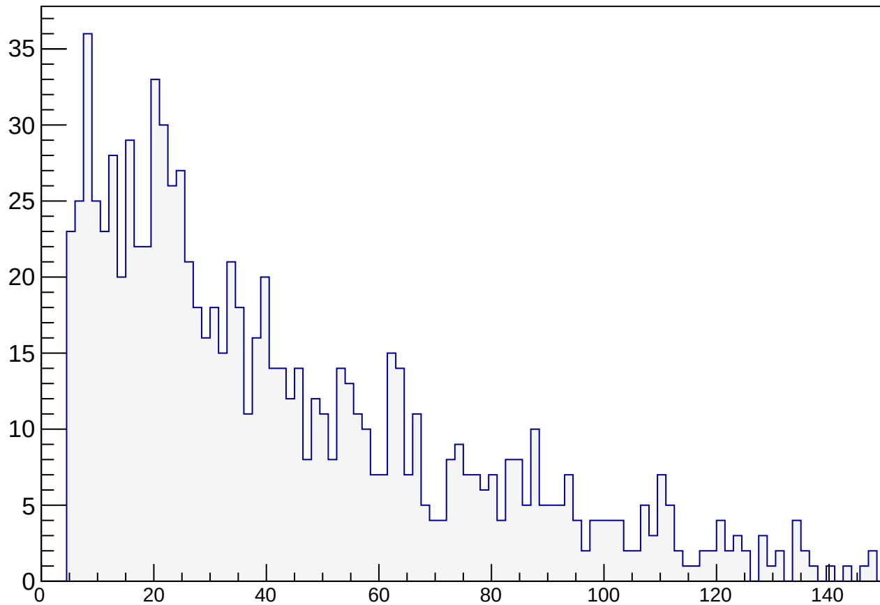
IXY_fittedDimuon_bSpot_sig
