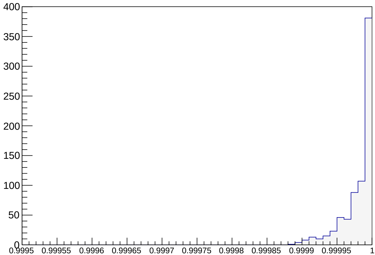
cosAngleModBsBSpot2D
