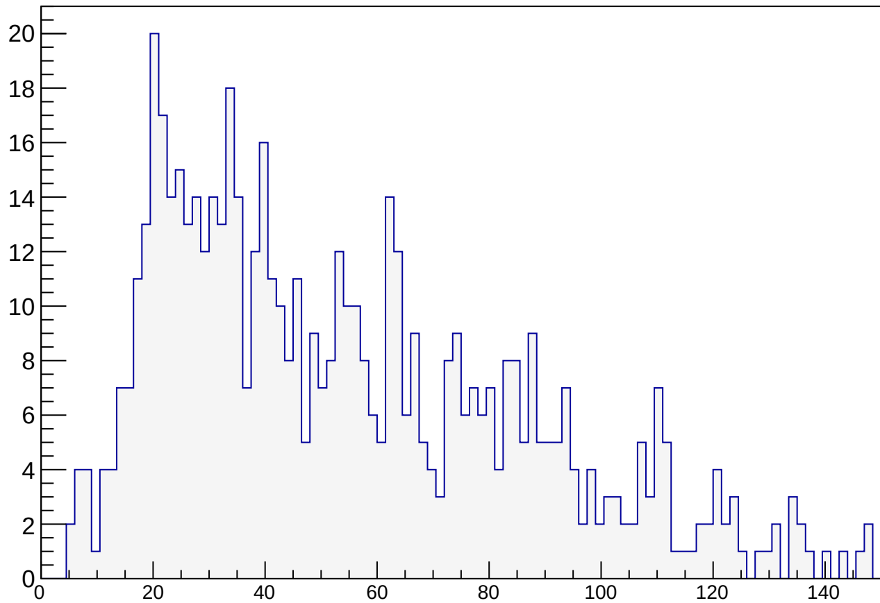
IXY_fittedDimuon_bSpot_sig
