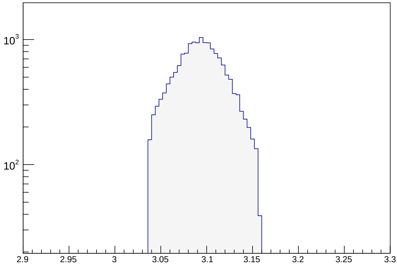
fittedDimuonMass
