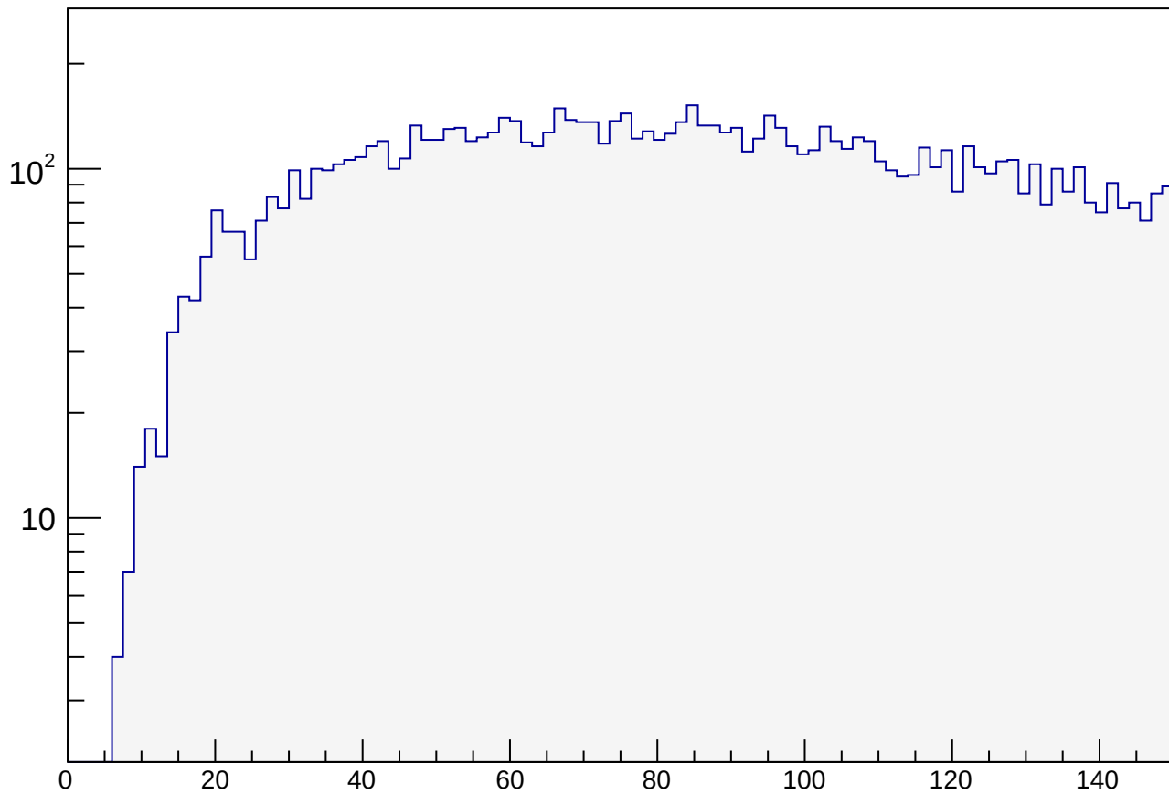
IXY_fittedDimuon_bSpot_sig
