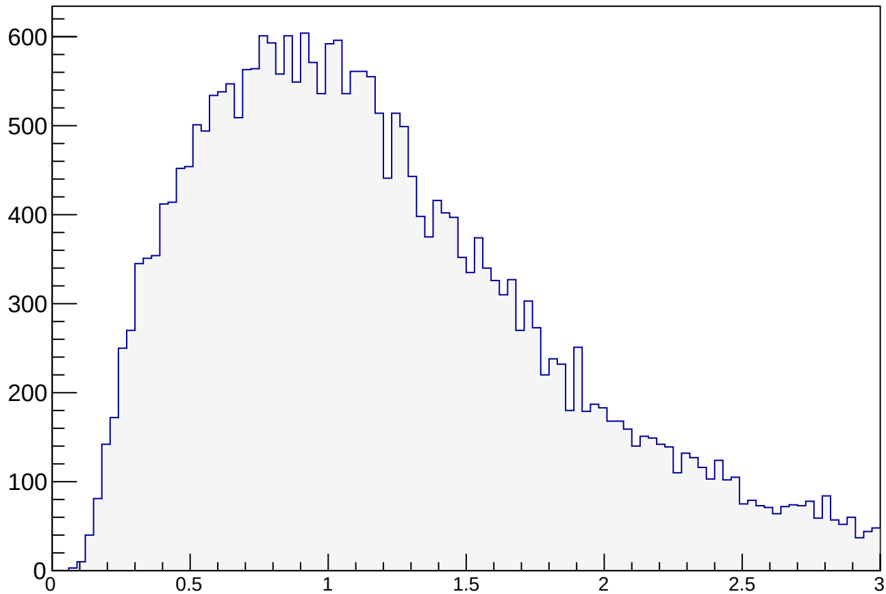
IXY_fittedDimuon_bSpot
