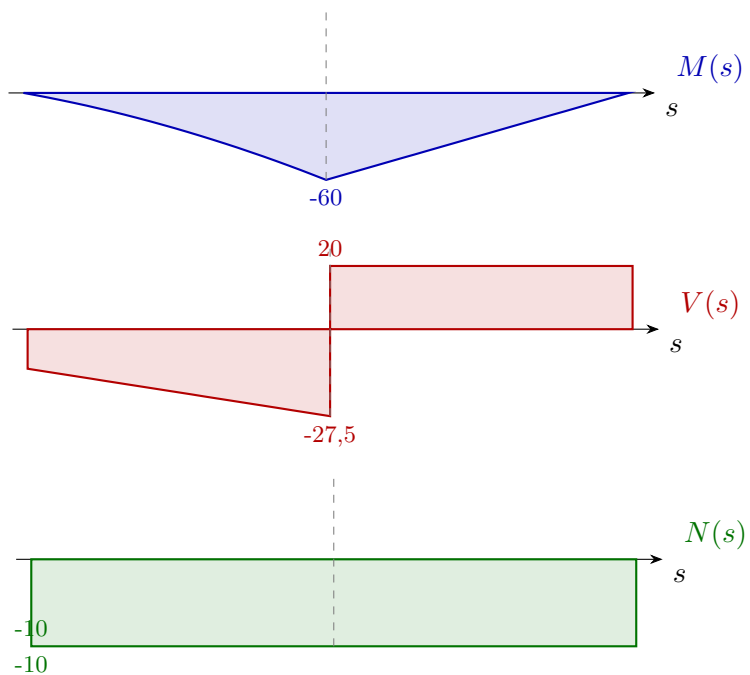
Biegeträger 2
