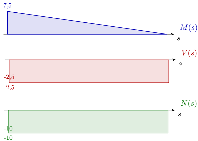
Biegeträger 1
