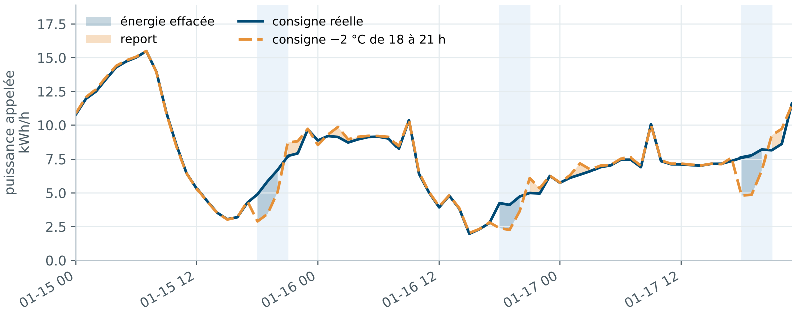
Bâtiment 185746 — trois jours de janvier, avec et sans effacement
