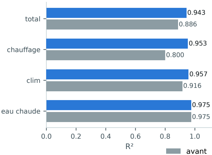
Modèle annuel — LightGBM
