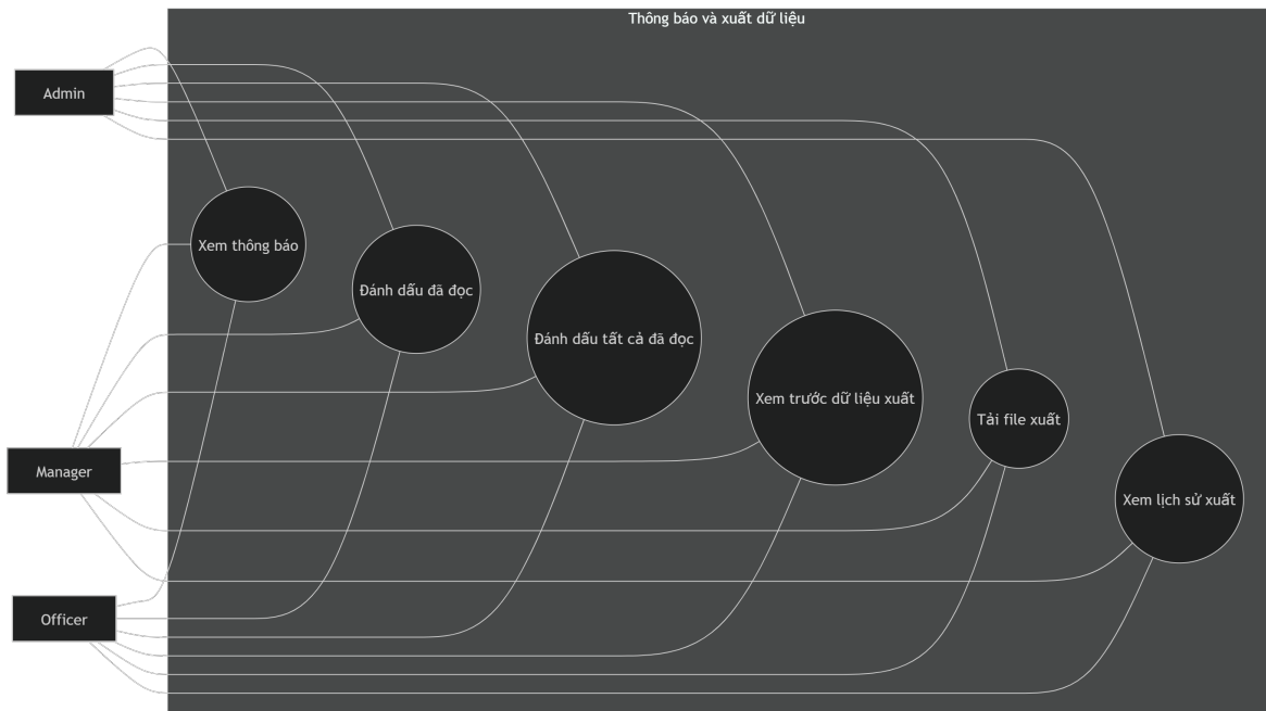
Hình 2.8: Biểu đồ use case phân rã nhóm thông báo và xuất dữ liệu
