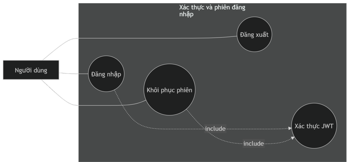
Hình 2.2: Biểu đồ use case phân rã nhóm xác thực
