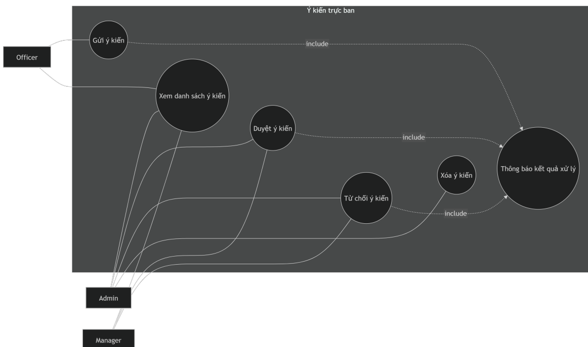
Hình 2.7: Biểu đồ use case phân rã nhóm ý kiến trực ban
