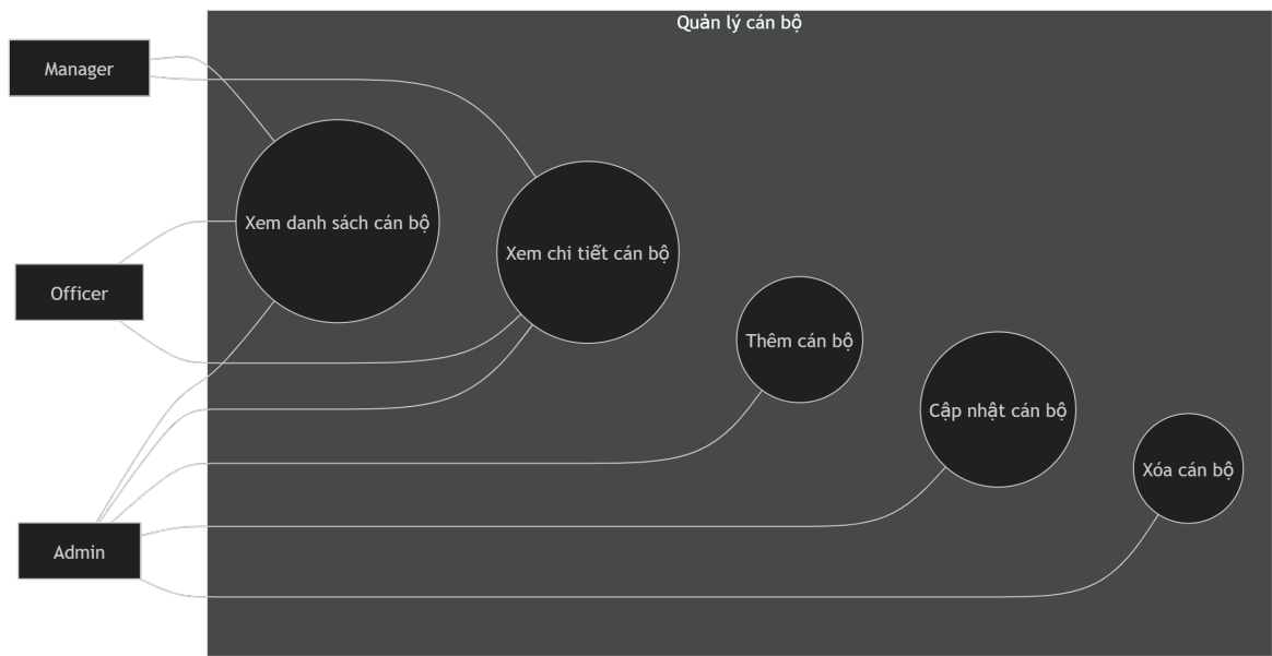
Hình 2.3: Biểu đồ use case phân rã nhóm quản lý cán bộ
