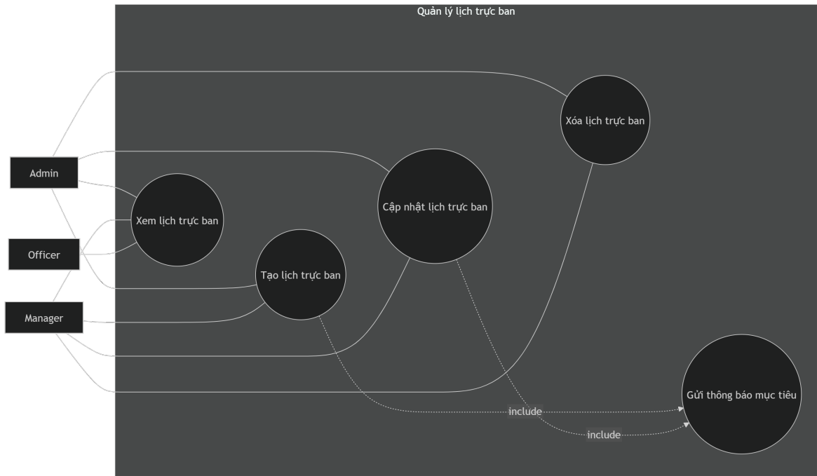
Hình 2.5: Biểu đồ use case phân rã nhóm lịch trực ban
