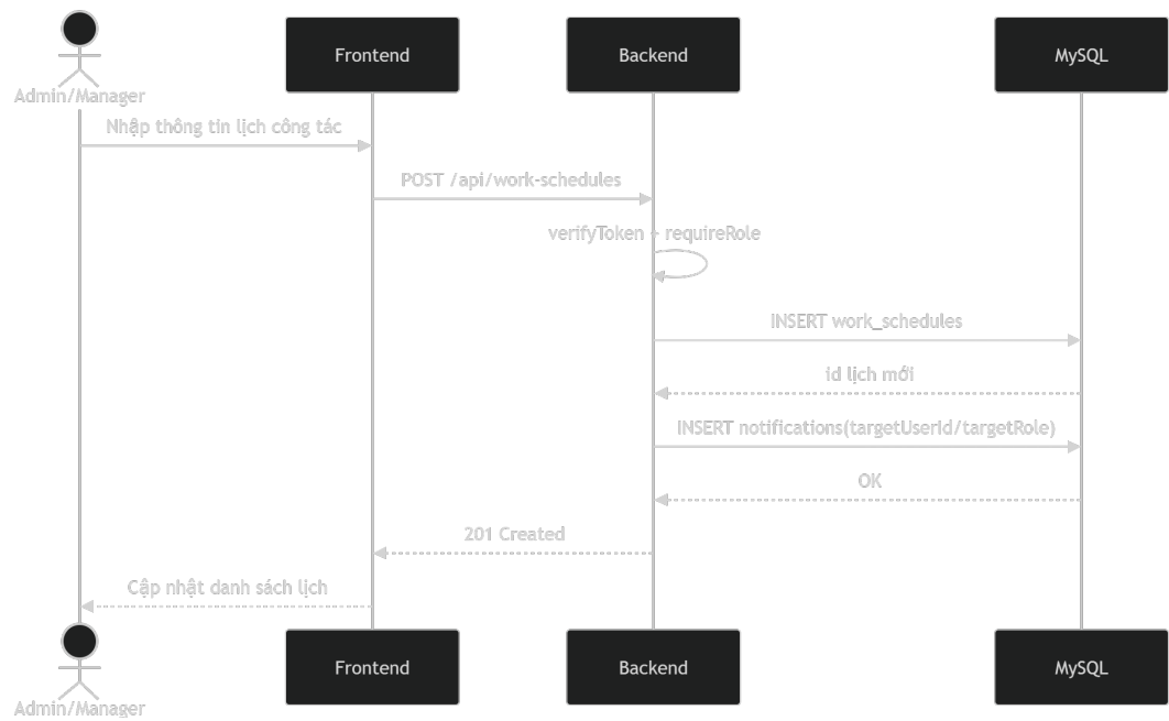
Hình 4.5: Biểu đồ trình tự use case tạo lịch công tác
