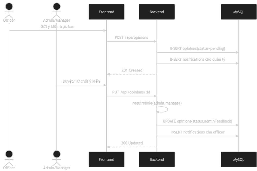
Hình 4.6: Biểu đồ trình tự use case ý kiến trực ban
