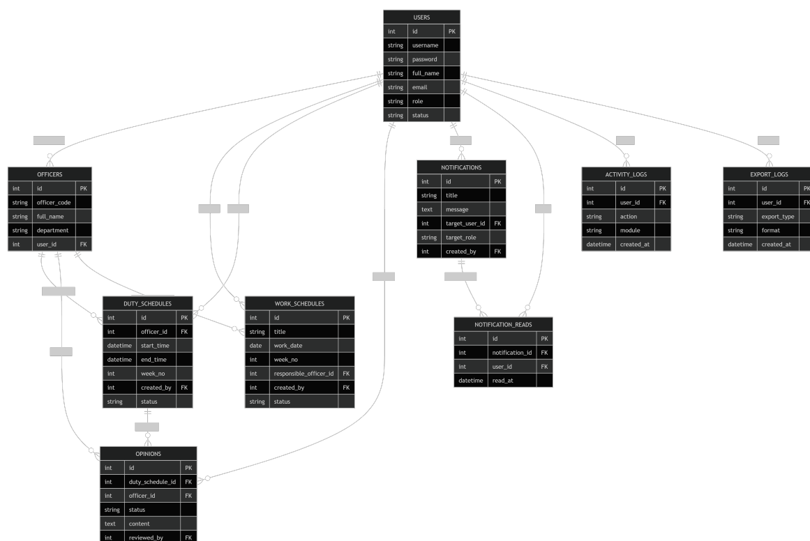
Hình 5.1: Biểu đồ ERD hệ thống
