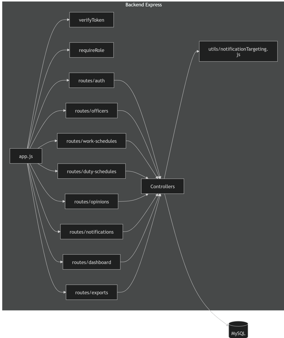
Hình 4.3: Biểu đồ thành phần backend
