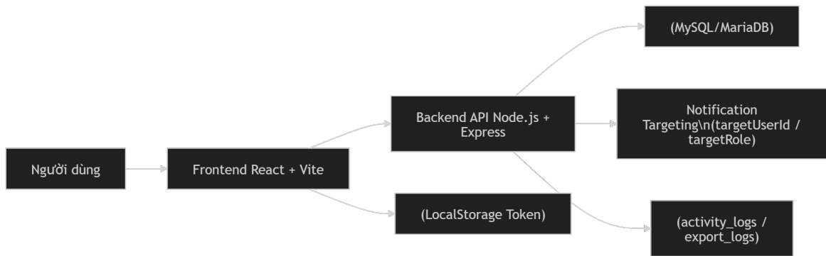
Hình 4.1: Biểu đồ kiến trúc tổng thể
