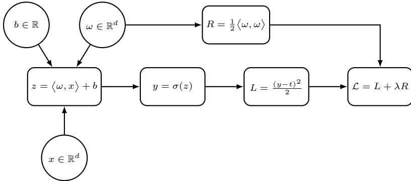
Рис. С2.2: Граф вычислений: логистическая регрессия с MSE и L_2 -регуляризацией.
