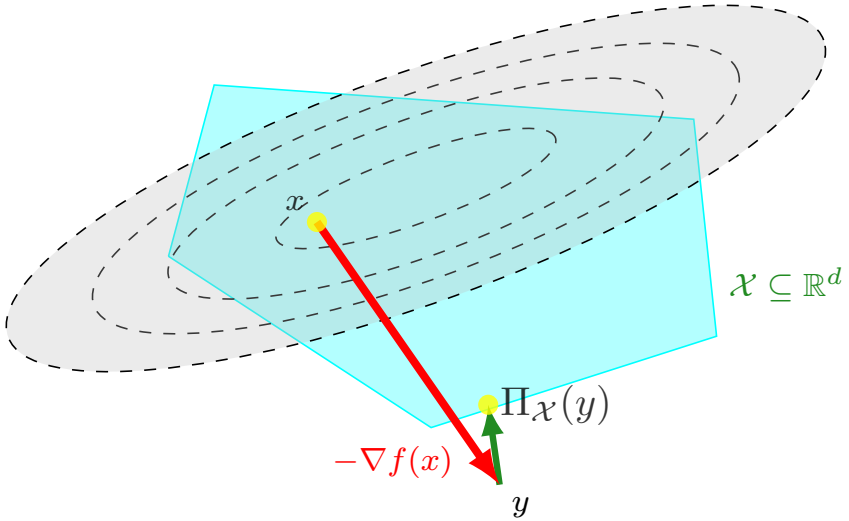
Рис. Л9.3: Проекция на множество
