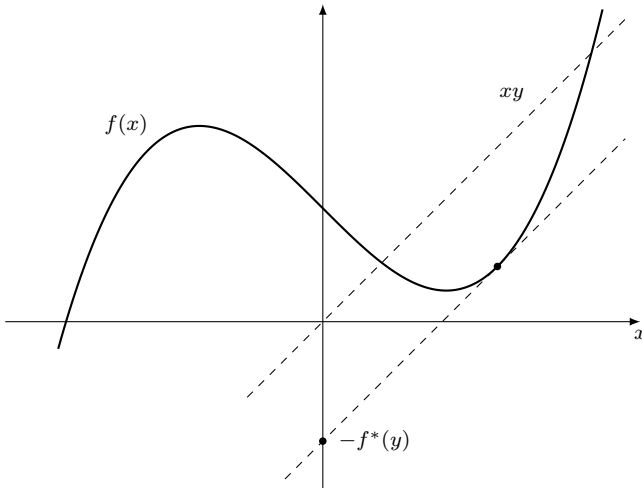
Рис. С6.1: Зазор показан пунктирными линиями. Если f(x) дифференцируема, то пунктирная линия касается f в точке x , где f'(x) = y .
