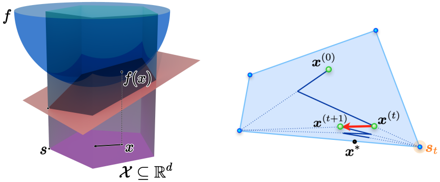
Рис. Л9.4: Шаг Франк-Вульфа
