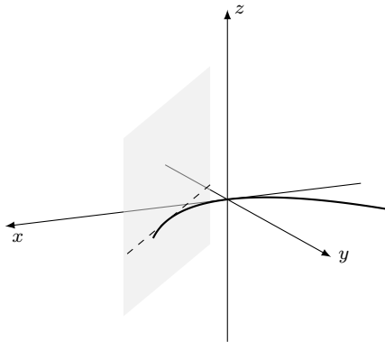
Рис. C5.1: Пример, когда субдифференциал — неограниченное множество.
