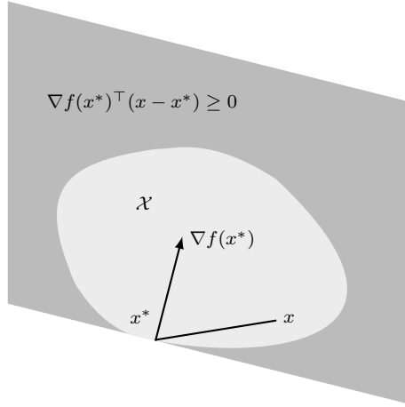
Рис. Л9.2: Иллюстрация оптимального условия из Теоремы Л9.1.
