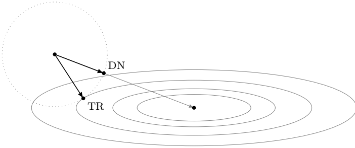
Рис. Л7.3: Вытянутые уровни f ; доверительный круг снаружи, касание внешнего уровня; шаг TR к касанию, демпфированный Ньютон — к центру.
