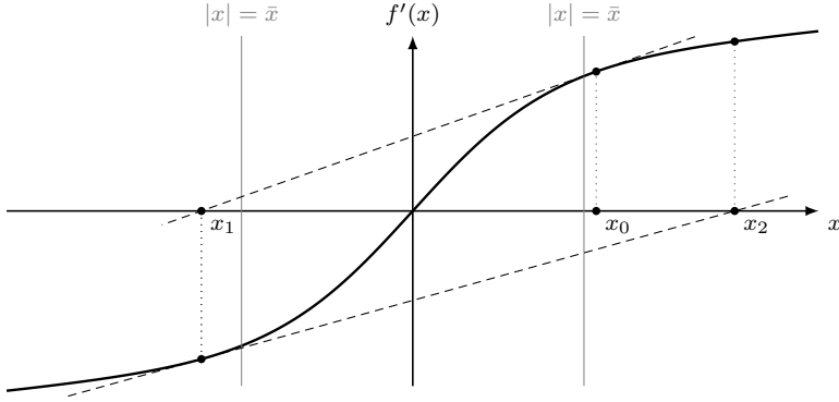
Рис. Л7.2: Метод Ньютона для минимума f(x) = \frac{x^2}{2} + 10 \log \cosh x : геометрия шагов на графике f'(x) . Можно заметить, что график очень похож на Л7.1
