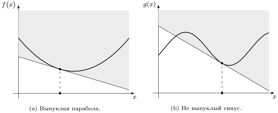
Рис. С4.4: Выпуклость через условие первого порядка.
