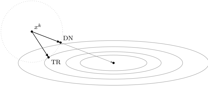
Рис. Л7.2: Линии уровня квадратичной модели m_k(p) , область доверия ограничена пунктиром, показаны шаги Trust-Region и демпфированного метода Ньютона.
