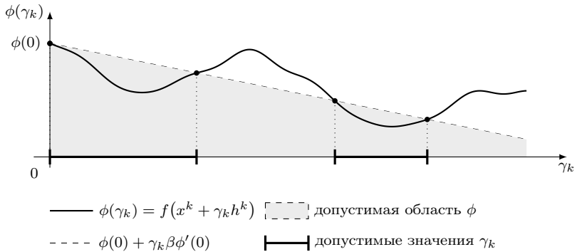
Рис. ЛЗ.3: Иллюстрация условия Армихо.
