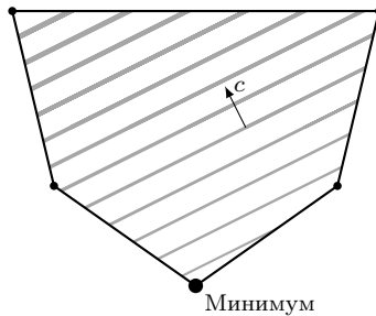
Рис. С11.1: Допустимое множество (штриховка) и ограничивающие прямые. Уровни c^\top x параллельны штрихам.
