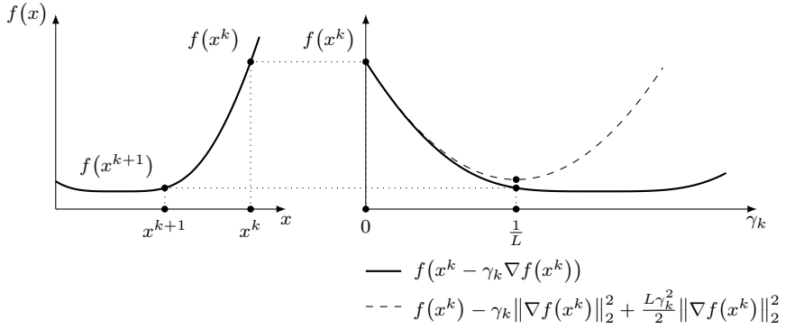
Рис. 13.2: Иллюстрация шага градиентного спуска с оптимальным \gamma_k = \frac{1}{L} .
