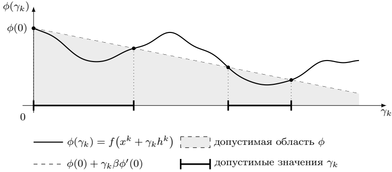
Рис. ЛЗ.3: Иллюстрация правила Армихо.
