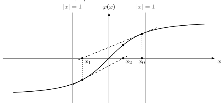
Рис. Л7.1: Сходимость в зависимости от начального приближения.
