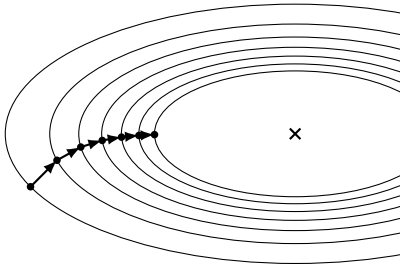
(a) Градиентный спуск.
