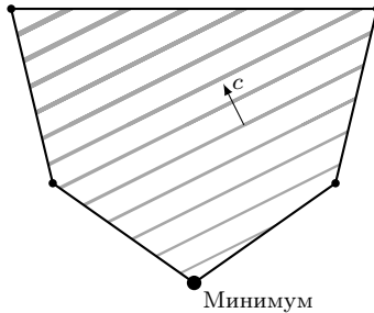
Рис. С10.1: Допустимое множество (штриховка) и ограничивающие прямые. Уровни c^\top x параллельны штрихам.
