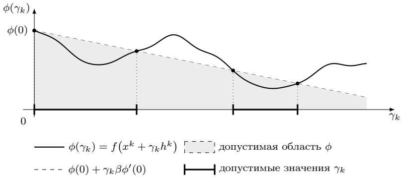
Рис. ЛЗ.3: Иллюстрация условия Армихо.
