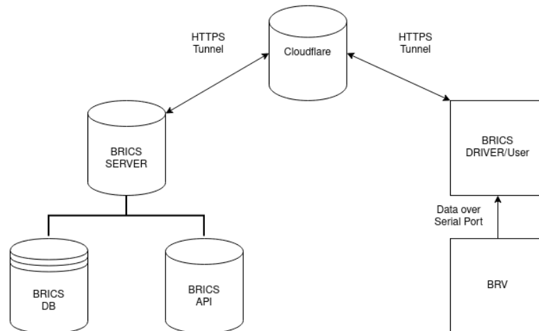
Rysunek 4.1: Uproszczony diagram transmisji danych wewnątrz projektu
