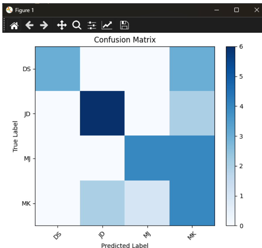
Rysunek 6.2: Wykres przedstawiający macierz konfuzji klasyfikatora danych surowych dla 4 klas
