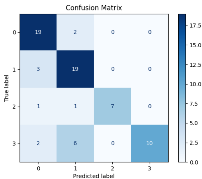
Rysunek 6.4: Wykres przedstawiający macierz konfuzji klasyfikatora NN dla 4 klas
