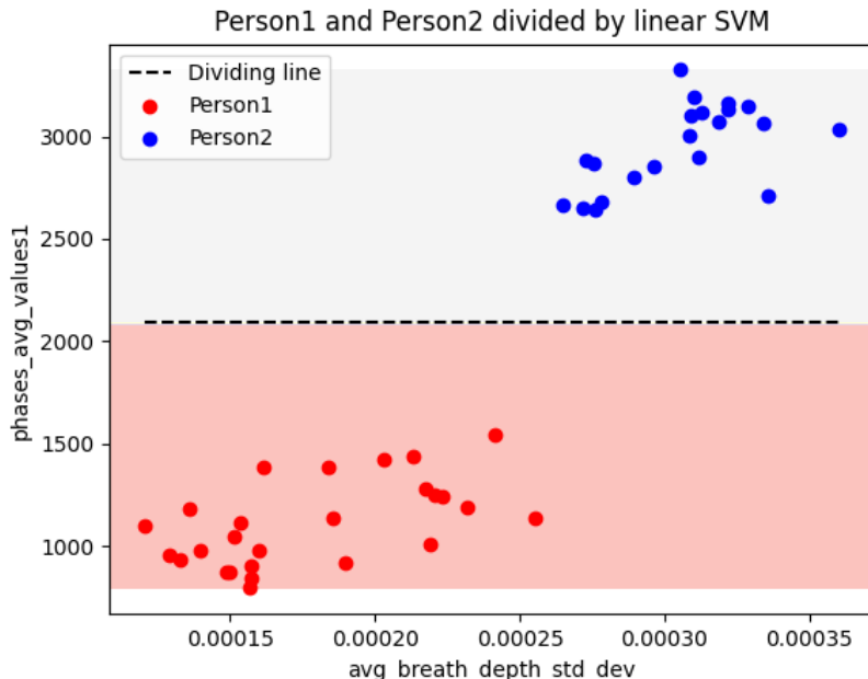
Rysunek 6.3: Wykres przedstawiający binarny klasyfikator SVM rozdzielający dwie klasy
